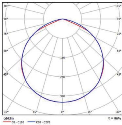
Óptica asimétrica
