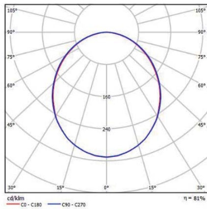
Óptica transparente
