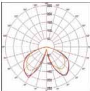
Ref. 3330 Dural con óptica simétrica 170°
