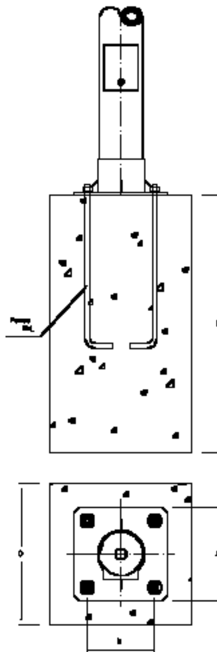
Detalle de la cimentación
