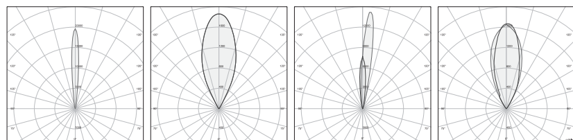
Simétrica 11° Simétrica 48° Asimétrica 11° Asimétrica 48°
