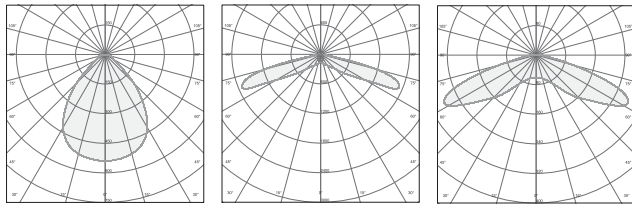
- Estándar R Ruta evacuación A Antipánico
