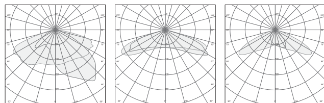
3405 Asimétrica extensiva 3406 Simétrica extensiva 3407 Asimétrica longitudinal
