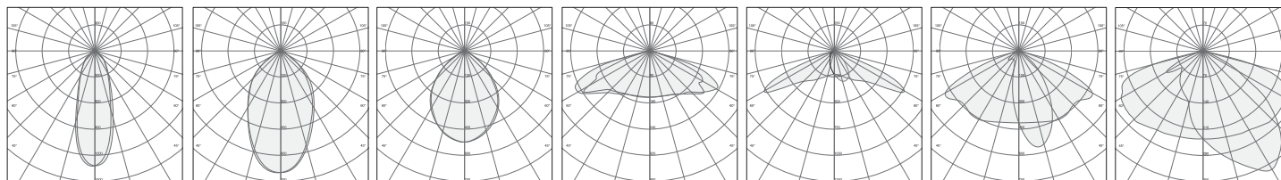
3414 Simétrica intensiva 31° 3415 Simétrica media 56° 3416 Simétrica extensiva 81° 3412 Simétrica extensiva 3413 Asimétrica longitudinal 3408 Asimétrica intensiva 3409 Asimétrica media
