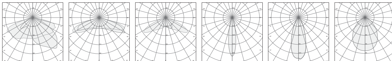
3405 Asimétrica extensiva 3406 Simétrica extensiva 160° 3407 Asimétrica longitudinal 3414 Simétrica intensiva 27° 3415 Simétrica media 56° 3416 Simétrica extensiva 85°
