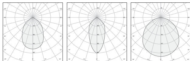
Sin óptica secundaria 90°
