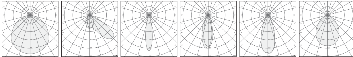
Sin óptica secundaria 120° 3501 Simétrica frontal 3502 Simétrica intensiva 22° 3503 Simétrica media 32° 3504 Simétrica media 3505 Simétrica extensiva
