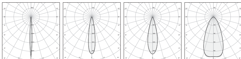
0 7° 1 14° 2 29° 3 46°
