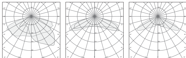
3405 Asimétrica extensiva
