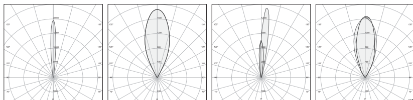
Simétrica 11°
