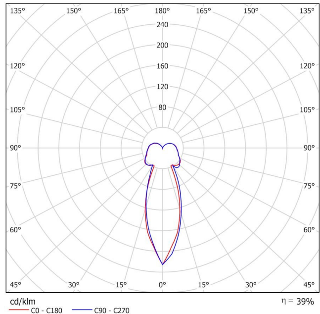
Ura con cierre opal - Óptica simétrica 150°
