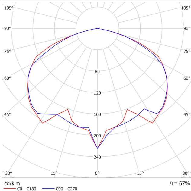
Ura sin cierre - Óptica simétrica 150°
