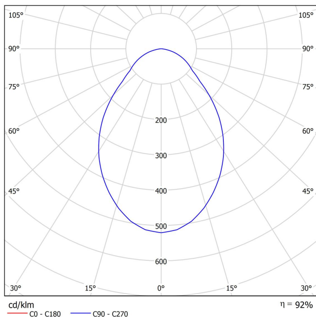
100W Óptica 80° - 80° Optics
