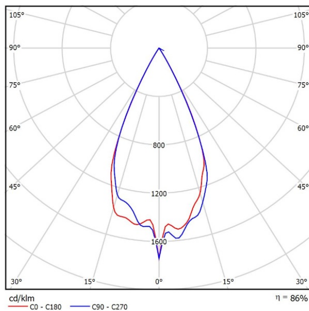
100W Óptica 48° - 48° Optics
