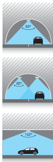
Esdium Tunnel M2 - 300w - Horizontal - Óptica asimétrica 2 lados Esdium Tunnel M2 - 300w - Horizontal - Asymmetric optics 2 sides
