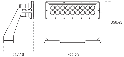
Esidium Pro LED M1 - Horizontal
