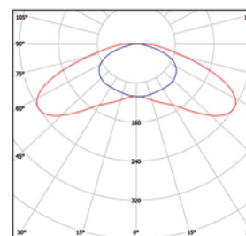
Ref. 3407 Óptica asimétrica de 150° Asymmetrical optical 150°
