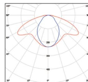
Ref. 3407 Óptica asimétrica de 80° Asymmetrical optical 80°
