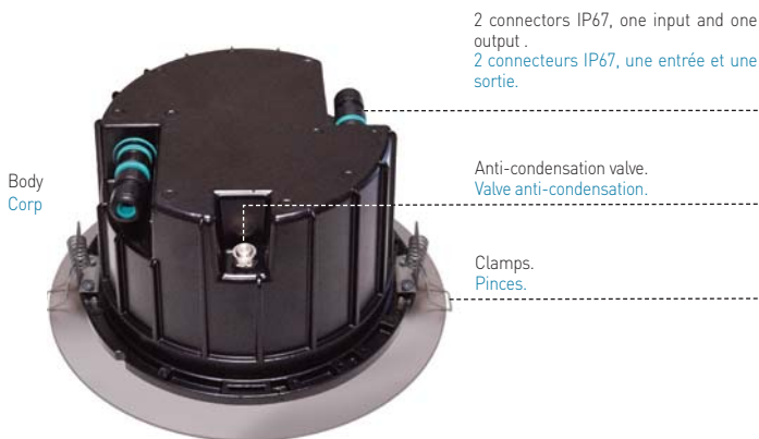
Ref. 51C3 Recessed auxiliary box on site. Boîte auxiliaire encastré sur place.
