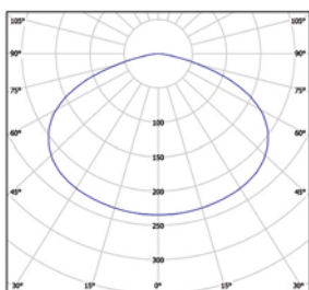
Symmetric optical 150° Optique symétrique 150°
