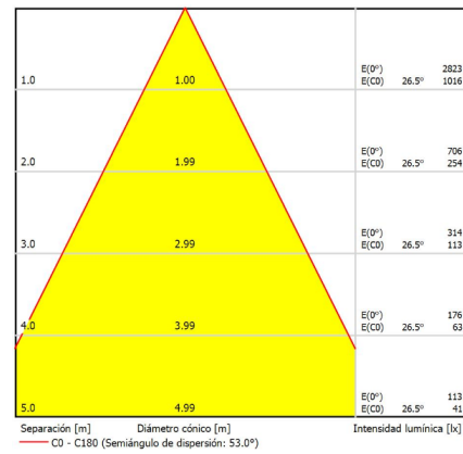
31W Óptica 54° / 54° Optics
