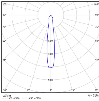
13W Óptica 16° / 16° Optics
