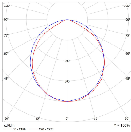
Difusor transparente
