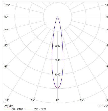
Óptica simétrica media 32° / Medium symmetric optics 32°
