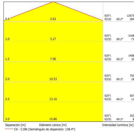
150W 3000K Óptica 150°/Optic 150°
