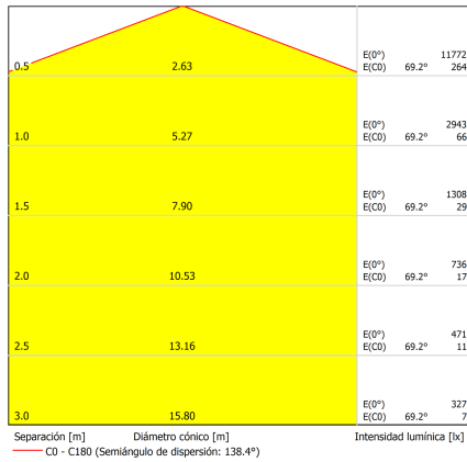
150W 3000K Óptica 80°/Optic 80°
