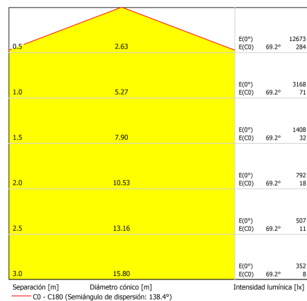
150W 4000K Óptica 150°/Optic 150°
