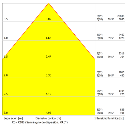
150W 4000K Óptica 80°/Optic 80°
