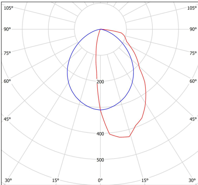
cd/klm \eta = 64\% — C0 - C180 — C90 - C270
