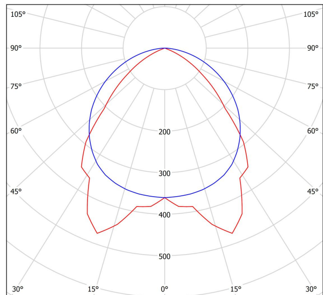
2x28W Reflector simétrico / Symmetric reflector
